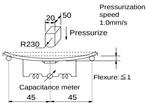
Fig.2 (in:mm)
