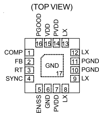
VQFN-16L 4x4
