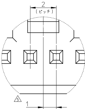
詳細図1 Scale 10:1
