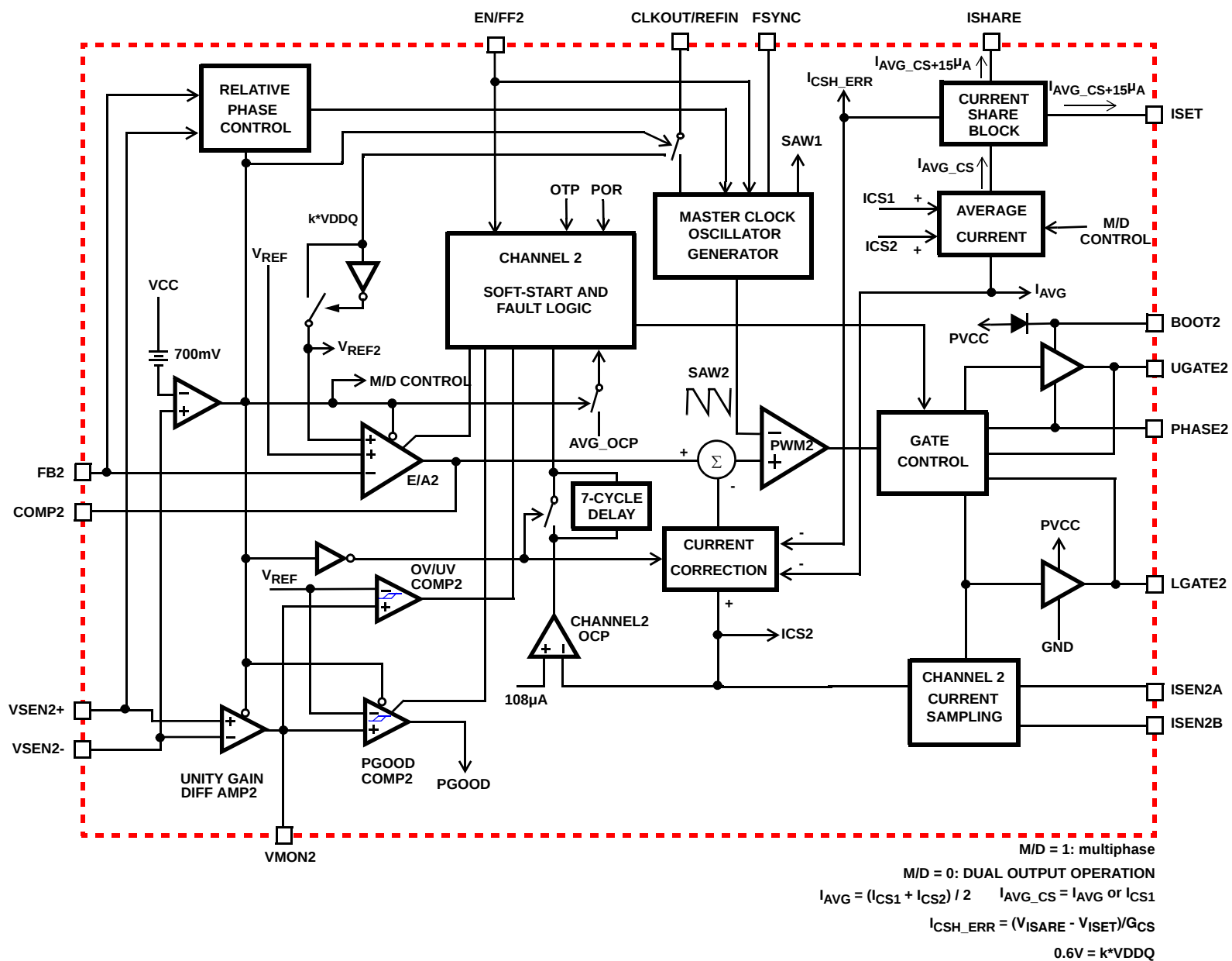
FIGURE 2. CHANNEL/PHASE 2 (VTT)
