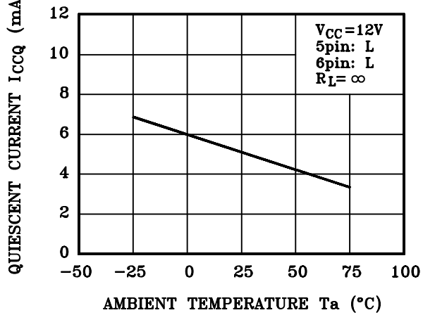
I_{CCQ} - T_a
