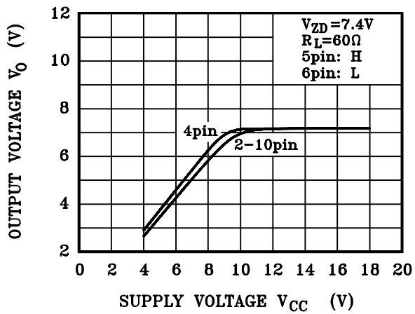
V_O - V_{CC}
