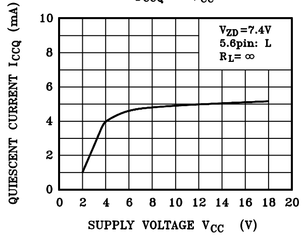
I_{CCQ} - V_{CC}
