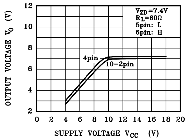
V_O - V_{CC}
