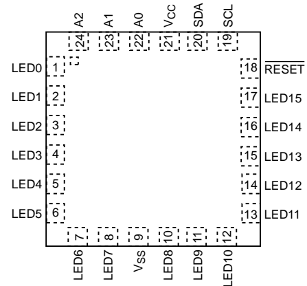
TQFN (HV6)
