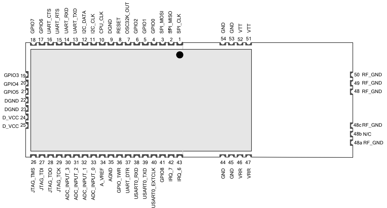
ZDM-A1281-PN0 Pinout
