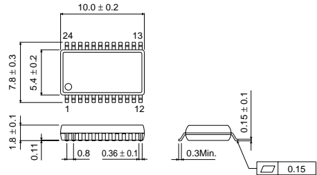
SSOP-A24
