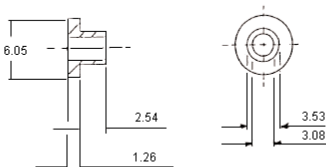
Dimensions : Millimetres
