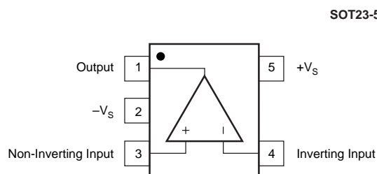
SOT23-5
