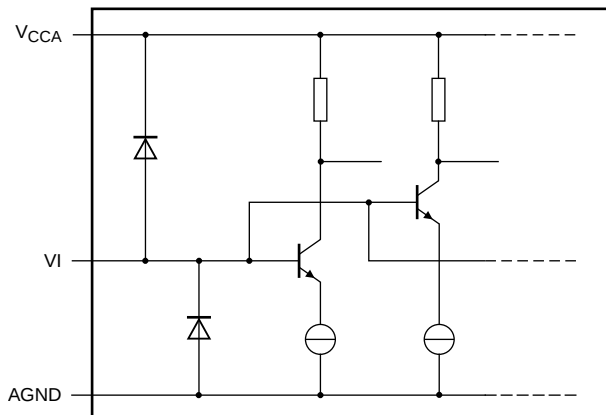
Fig 10. Analog inputs
