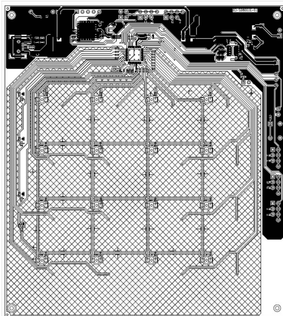
Figure 19. Bottom Layer
