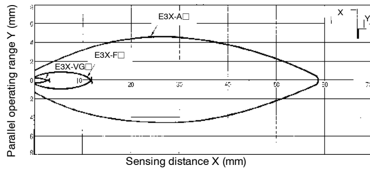
E32-D14L with E3X-A, E3X-F and E3X-VG amplifiers
