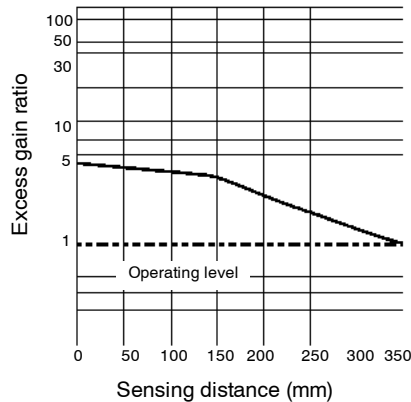
E32-UTAT1-3F with E3X-A11 amplifier
