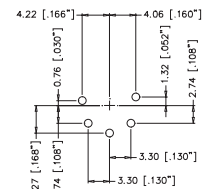
AC5M*ZV
