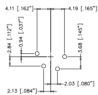
AC4F*ZV
