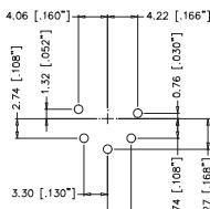
AC5F*ZV
