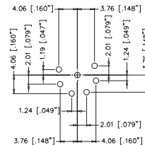
AC7M*ZV
