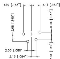
AC4M*ZV
