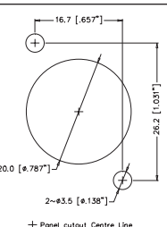
AC-PDN-34-XXX
