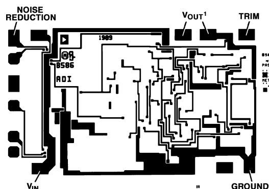
DIE LAYOUT
