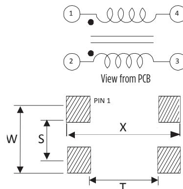
SODLER PAD(mm)
