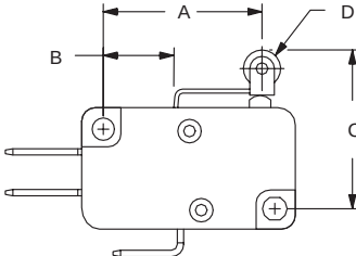
FIG. 1 Lever Roller
