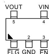
SOT-23-5
