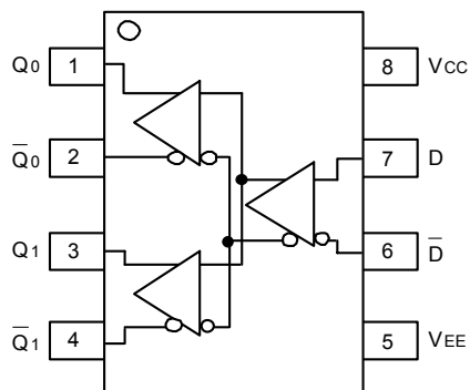
8-Pin SOIC (Z8-1)
