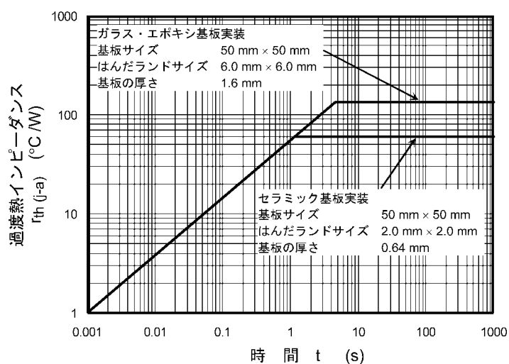
図 10.6 r_{th(j-a)} - t
