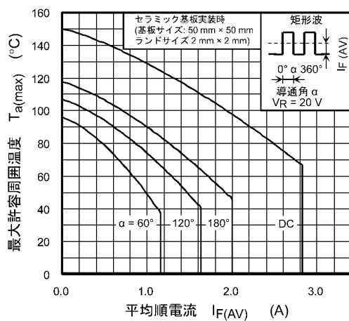
図 10.3 T_{a(max)} - I_{F(AV)}
