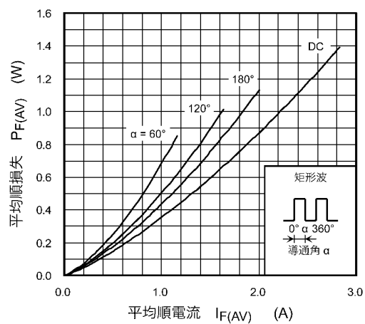
図 10.2 P_{F(AV)} - I_{F(AV)}
