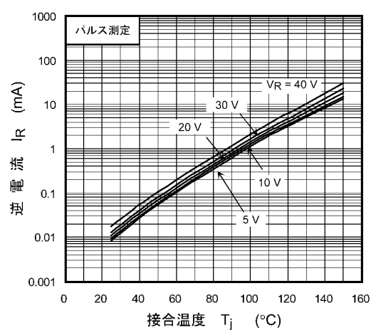
図 10.8 I_R - T_j
