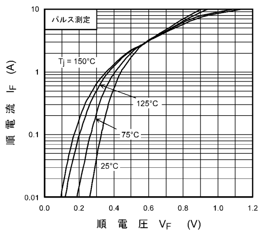
図 10.1 I_F - V_F
