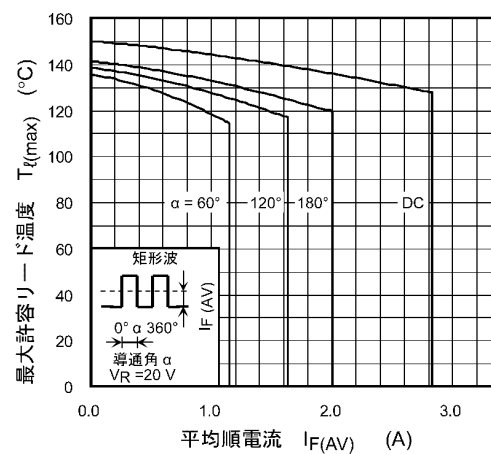
図 10.4 T_{l(max)} - I_{F(AV)}
