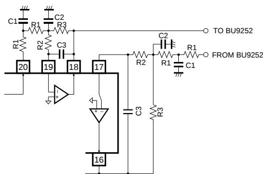
Fig. 4 LPF
