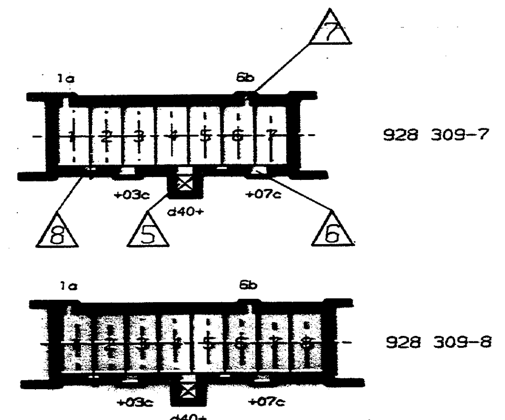
928309-8 8 natur 49 35 40 927740-8 927740-7 928151-7 928...-6 828353-7 928309-7 7 natur 44 30 35 927740-7 928151-7 928...-6 828353-7 Bestell-Nr. Polzahl Farbe Maß W Maß X Maß Y Stand.Timer Geh. AMP-MULTIFITTING conn. passende Gegenstecker ZEICHNUNG GÜLTIG AB XX.YY. AMP AMP DEUTSCHLAND G.m.b.H. Langen b.Ffm., West Germany BEZUGSNAME 7/8POL.FASTIN-ON GEHÄUSE, Raster 5mm siehe Tabelle - - - PAS.6 UL94-V2 siehe Tabelle OBERFLÄCHE K BESTELL-NR. POS. STOCK BENENNUNG EINZELTEIL WERKSTOFF FARBE HÖCHT TOLERIERTE MASSE ± 0,2mm ± 1° FORMAT A1 ZEICHNUNGS-NR. 928 309 GRZ. 08.12.68 GEP. Schneiders SCHNAUDEL 08.12.68 MASSE S: (1;1) BLATT 1 VON 1 Körschner REV. β
