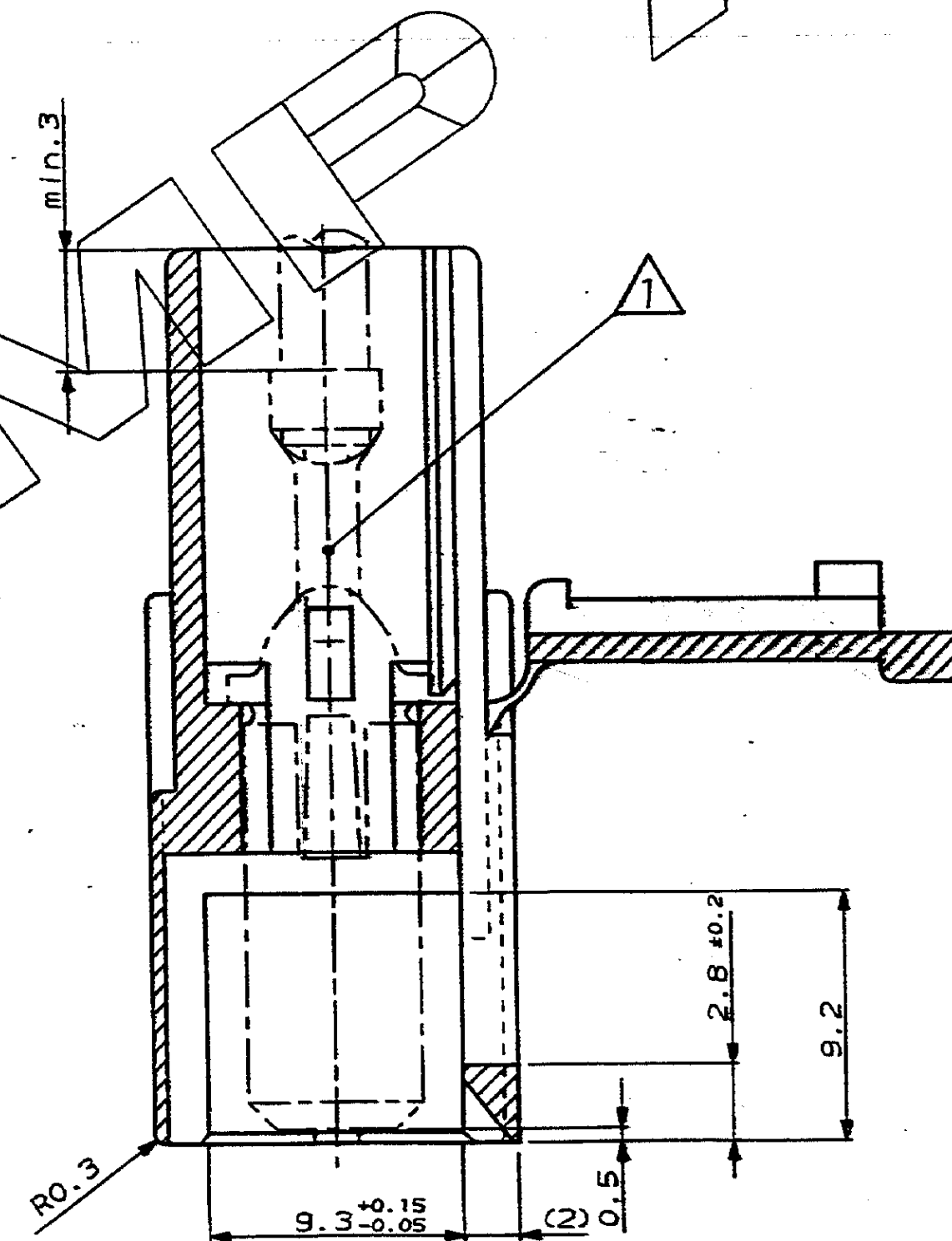
928309-8 8 natur 49 35 40 927740-8 927740-7 928151-7 928...-6 828353-7 928309-7 7 natur 44 30 35 927740-7 928151-7 928...-6 828353-7 Bestell-Nr. Polzahl Farbe Maß W Maß X Maß Y Stand.Timer Geh. AMP-MULTIFITTING conn. passende Gegenstecker ZEICHNUNG GÜLTIG AB XX.YY. AMP AMP DEUTSCHLAND G.m.b.H. Langen b.Ffm., West Germany BEZUGSNAME 7/8POL.FASTIN-ON GEHÄUSE, Raster 5mm siehe Tabelle - - - PAS.6 UL94-V2 siehe Tabelle OBERFLÄCHE K BESTELL-NR. POS. STOCK BENENNUNG EINZELTEIL WERKSTOFF FARBE HÖCHT TOLERIERTE MASSE ± 0,2mm ± 1° FORMAT A1 ZEICHNUNGS-NR. 928 309 GRZ. 08.12.68 GEP. Schneiders SCHNAUDEL 08.12.68 MASSE S: (1;1) BLATT 1 VON 1 Körschner REV. β
