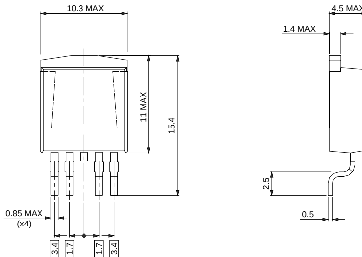
Fig.33. SOT426
