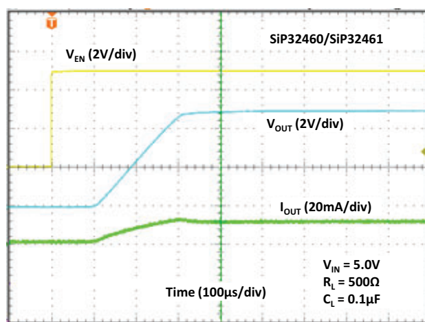
Fig. 25 - Turn-on Time
