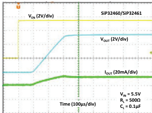
Fig. 29 - Turn-on Time
