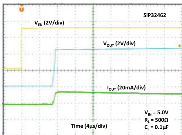
Fig. 33 - Turn-on Time
