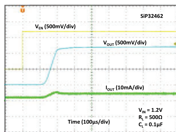
Fig. 30 - Turn-on Time
