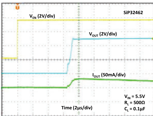
Fig. 31 - Turn-on Time
