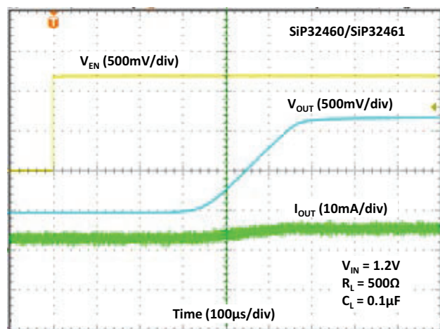
Fig. 24 - Turn-on Time
