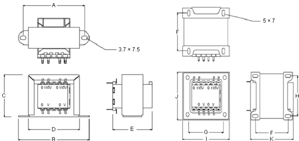
Dimensions : Millimetres
