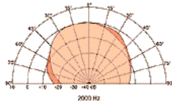
Abstrahlcharakteristik 2000 Hz
