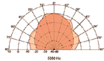
Abstrahlcharakteristik 5000 Hz
