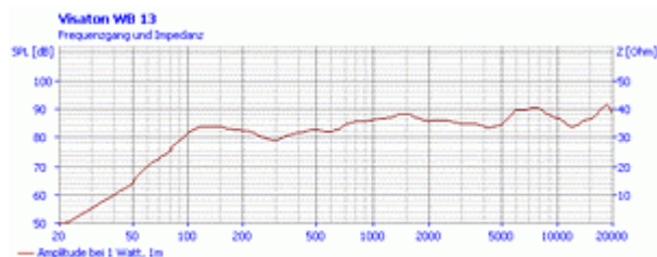
Amplitudenfrequenzgang
