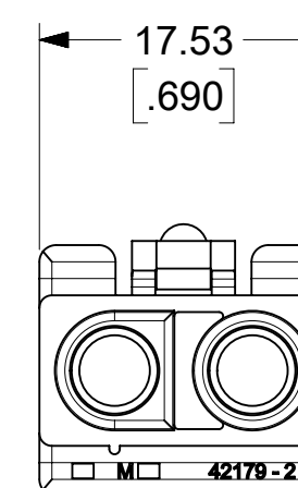
2 CIRCUIT RECEPTACLE
