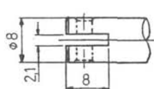
Ankerdetail
