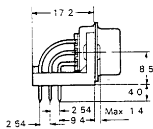
50 Way
