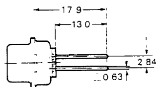
Wire Wrap
