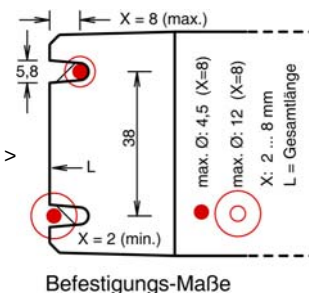
Befestigungs-Maße
