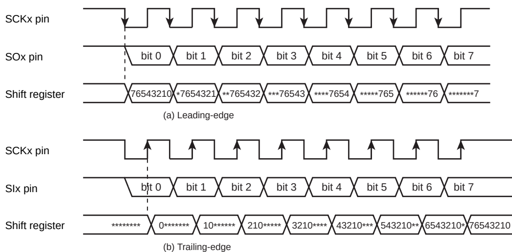
Figure 14-17 Shift Edge
