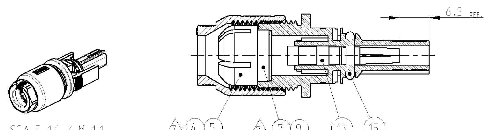
SECTION A-A SCHNITT A-A
