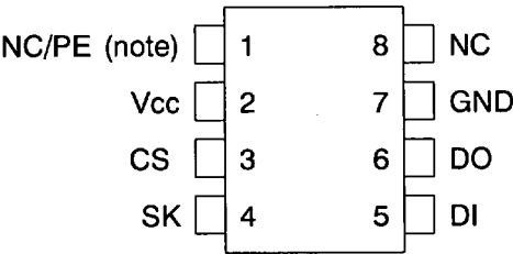
8pinSOP
