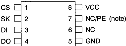
8pinTSSOP
