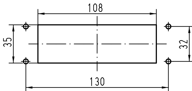
Montageausschnitt panel cut out 1:2
