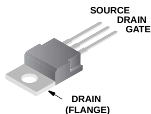
HUF76432P3
