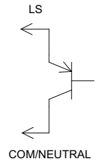
PNP O.C. TRANSISTOR OR (P) FET INPUT
