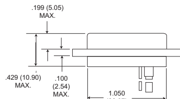
Receptacle
