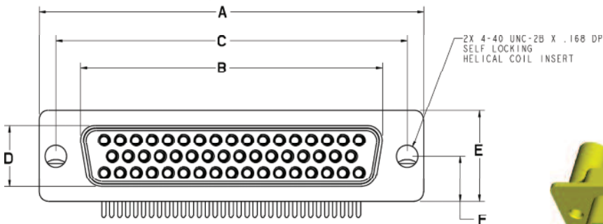
Receptacle - Socket
