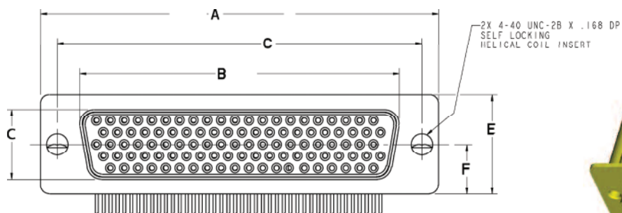
Receptacle - Socket
