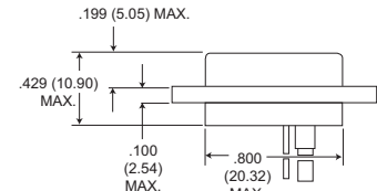
Receptacle
