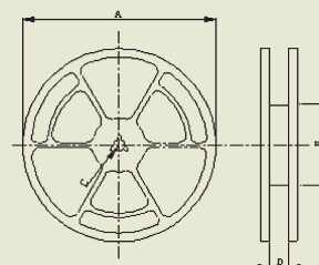
Reel Dimensions
