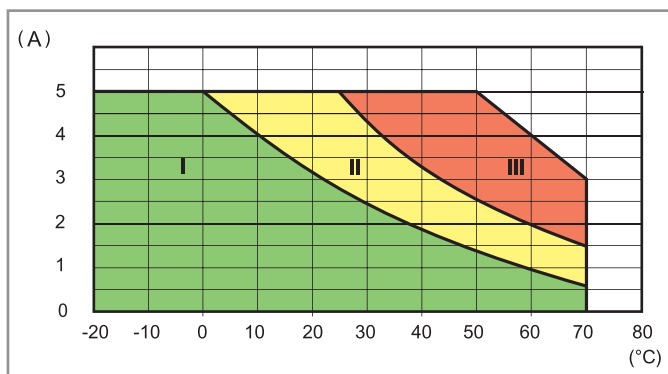
L77-1 Corrente RMS di uscita in funzione della temperatura ambiente 77.01.0.024.805x @ 32 V DC
