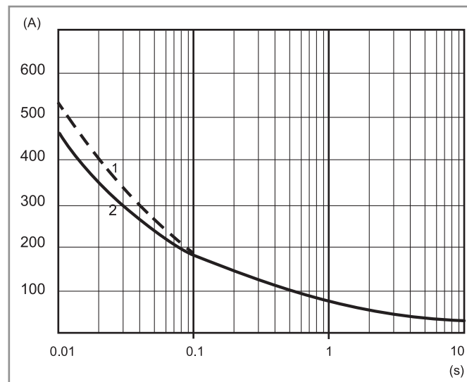
L77-5 Corrente di picco (AC) in funzione della durata 77.31.x.xxx.80xx
