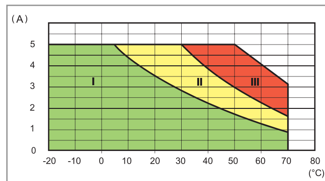
L77-2 Corrente RMS di uscita in funzione della temperatura ambiente 77.01.8.230.805x @ 265 V AC
