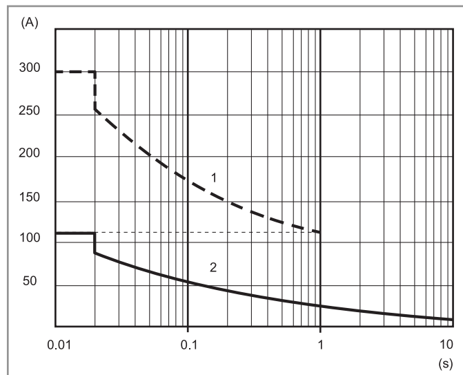
L77-3 Corrente di picco (AC) in funzione della durata 77.01.x.xxx.80xx
