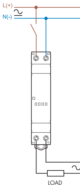
Connessione monofase (77.01)
