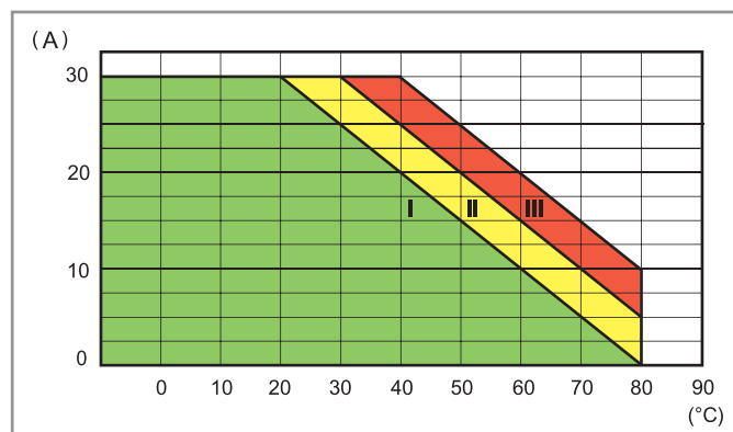
L77-4 Corrente RMS di uscita in funzione della temperatura ambiente 77.31.x.xxx.80xx
