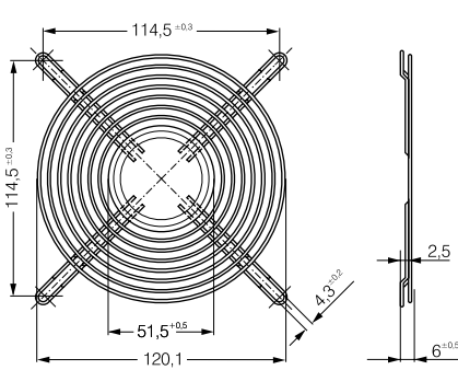
LZ35 Fan series 5200/5900
