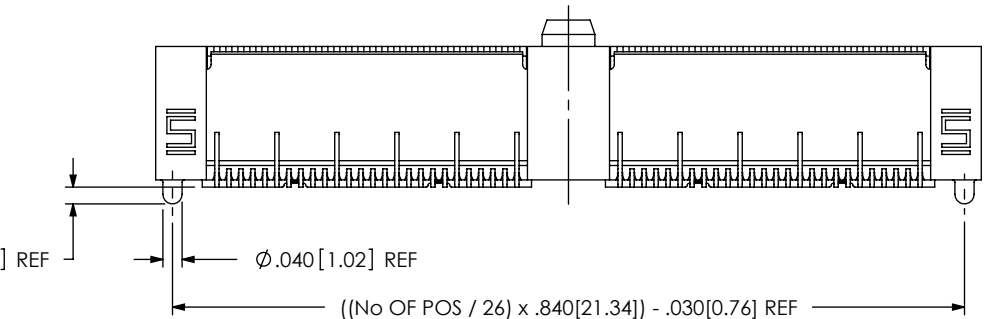
FIG 1 QFSS-052-04.25-X-D-A SHOWN
