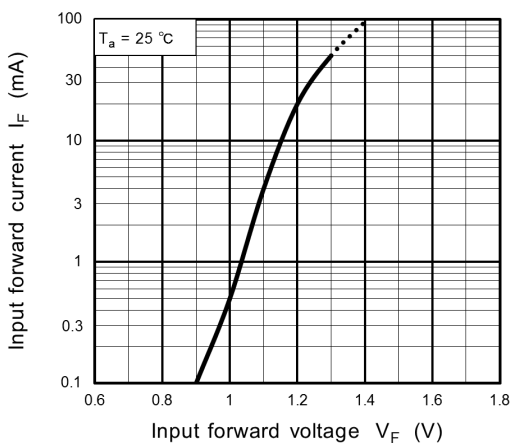
Fig. 12.4 I_F - V_F
