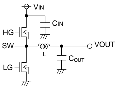
Fig.24 Input Capacitor
