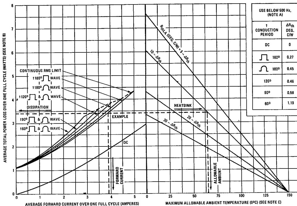
Fig. 8 - Thermal Nomogram
