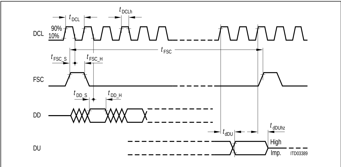
IOM®-2 Interface Timing
