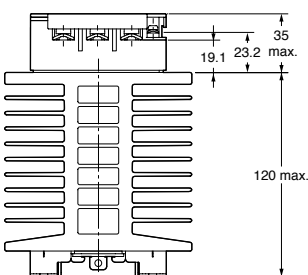
G3PE245B-3N
