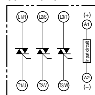
G3PE245B-3N
