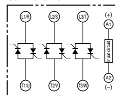
G3PE-545B-3N
