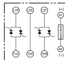
G3PE-545B-2N
