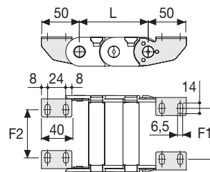
Bild. B Fixierung der Energieführungskette nach außen. (Bild B) Sie bitte die Einbauvarianten auf Seite 31.
