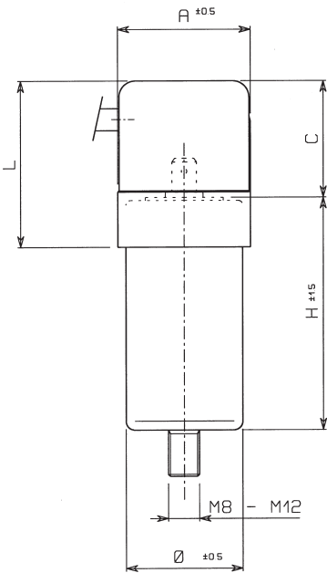
Fig. 6 Cappellotto plastico - IP55 con cavo plastico. Plastic cap - IP55 with twin cable.
