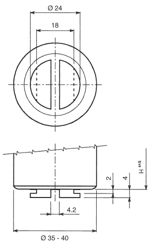
Fig. 5 Fissaggio rapido a slitta solo per dia 30-35-40 mm (su richiesta) Quick mounting slider for dia 30-35-40 mm only (on request)
