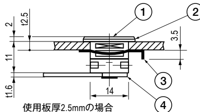
使用板厚2.5mmの場合 Mounting panel thickness of 2.5mm
