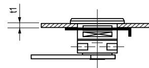
使用板厚1mmの場合 Mounting panel thickness of 1mm
