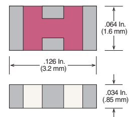
Case 18-2 (EIA 1206 / 3216)
