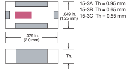
Case 15-3 (EIA 0805 / 2012)
