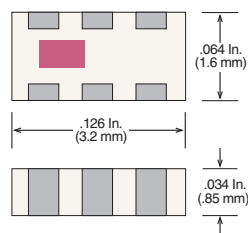
Case 18-1 (EIA 1206 / 3216)
